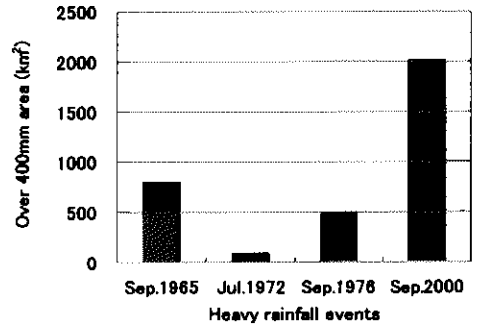
図7 主要豪雨時の2日降水量400mm以上の面積
