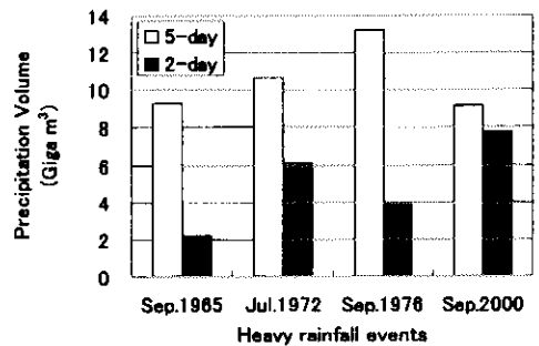
図8 主要豪雨時の降水総量
