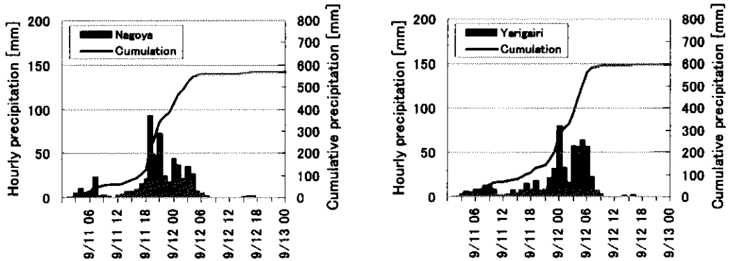
図4 名古屋・槍ヶ人の降水量の推移 (2000年9月11~12日)
