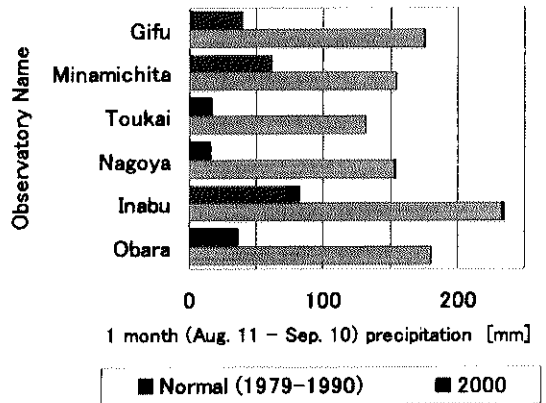
図3 主要観測所の8月11日～9月10日の降水量と準年平均値（1979～1990年の平均値）
