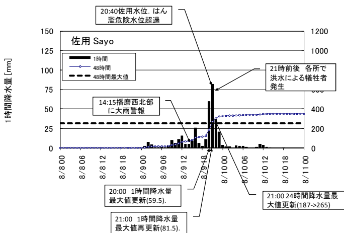
図 7 AMeDAS 佐用の降水量
