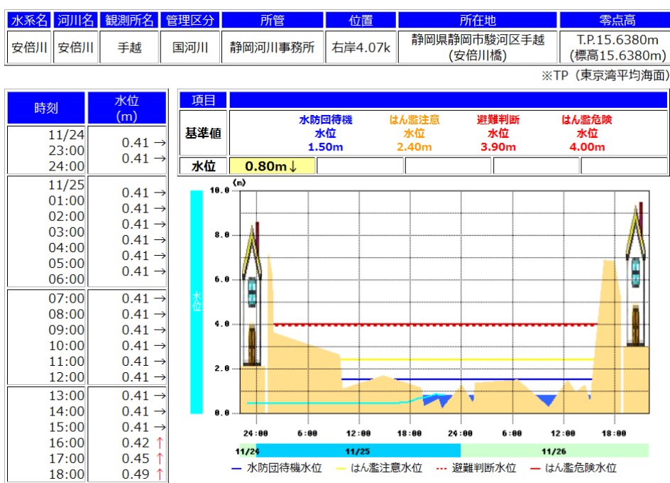
図 5 「川の防災情報」の水位情報表記の例
